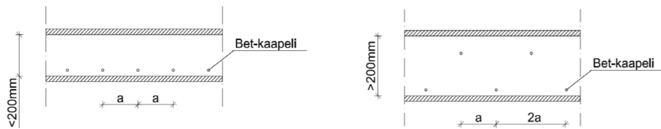
Betonin lämmityslangan sijoitus seinissä ja laatoissa, huomioitava myös reunoissa reunasilmukat
