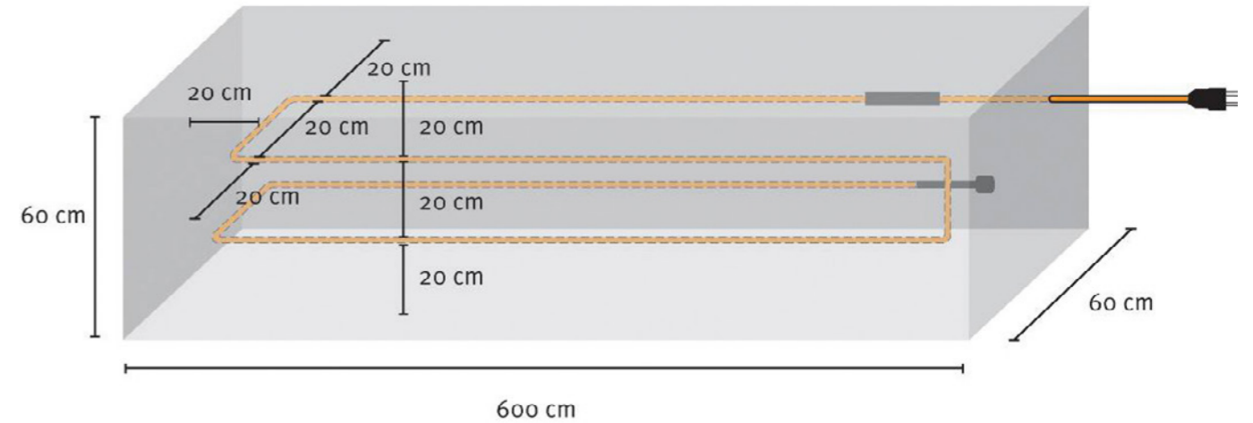
BET-lämmityskaapelin sijoittaminen rakenteeseen
