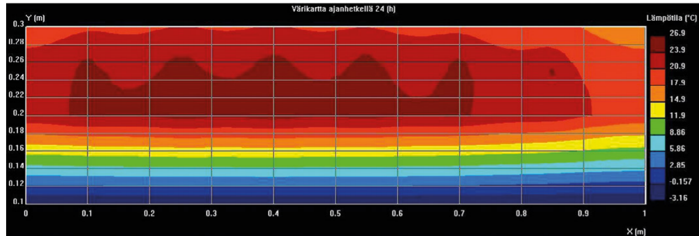
Esimerkki pintalaatan lämpöjakaumasta
