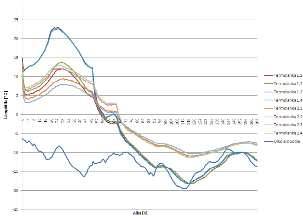
BET-lämmityskaapeilla lämmitettävän pintabetonilaatan lämmönkehitys seitsemän vuorokauden aikana.
