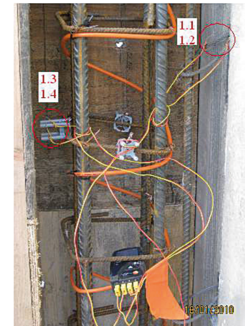
Termolankojen 2.1 – 2.4 sijoitus pilasterissa
