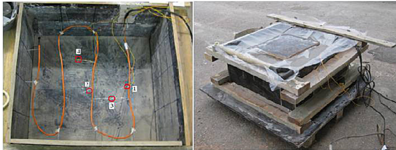
Lämmityskaapeloinnin sijoitus muottiin (vasemmalla); kappaleen säilytys pakkassäissä kaksi vuorokautta (oikealla).
