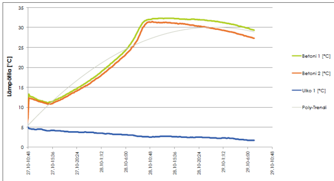
BET-lämmityskaapeilla lämmitettävän seinän lämmönkehitys kolmen vuorokauden aikana.
