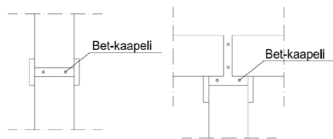
Betonilämmityskaapelin sijoitus päittäis- ja T-saumoissa
