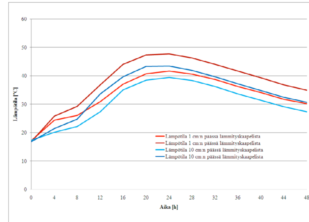
BET-lämmityskaapeleilla lämmitettävän betonikappaleen lämmönkehitys kahden vuorokauden aikana, ulkolämpötilan vaihdellissa -2 °C ja -8 °C välillä (lämmitysteho 580 W/m 3 ).
