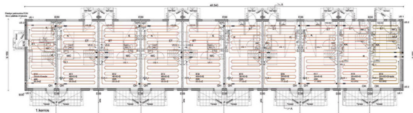
Esimerkkikohteen pohjakuva
